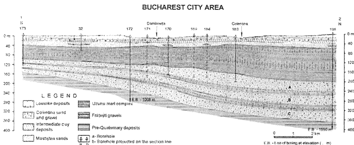
Fig. 4. Profil geologic N-S al zonei Bucureștiului
