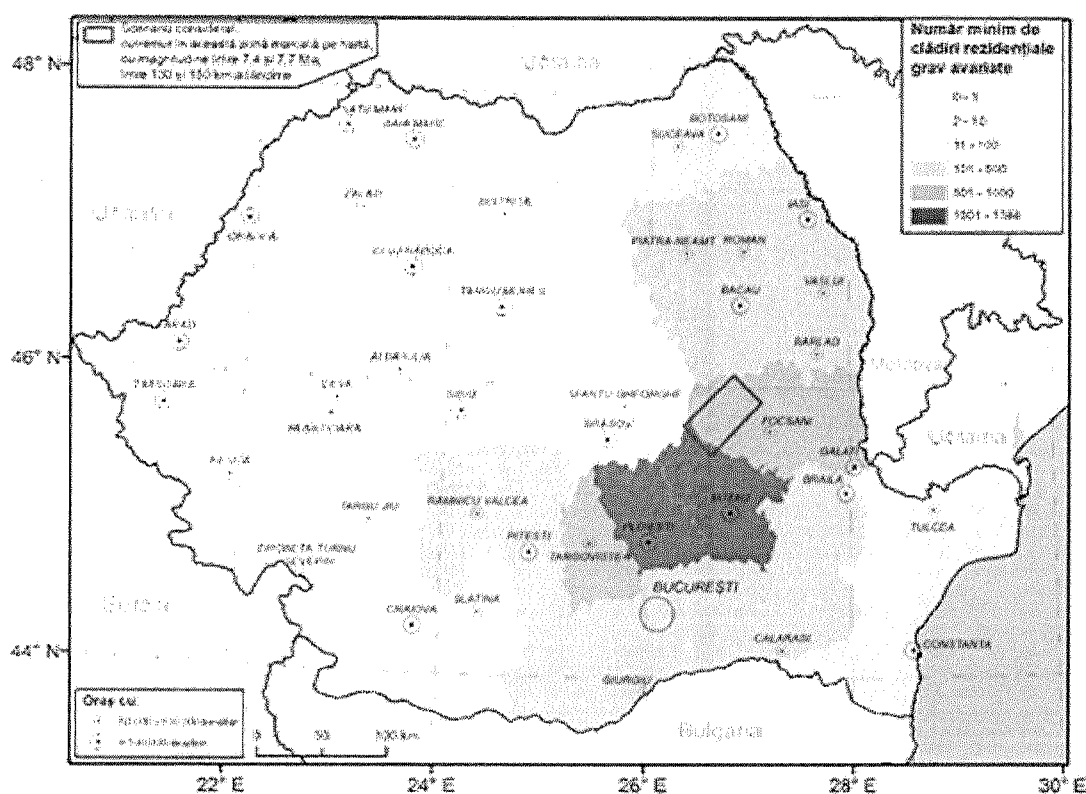
Fig. 22. Număr minim de clădiri rezidențiale grav avariate la nivel de județ, ca urmare a unui seism în zona marcată pe hartă, cu magnitudinea între 7,4 și 7,7 MW, la adâncimi între 130 și 150 km
