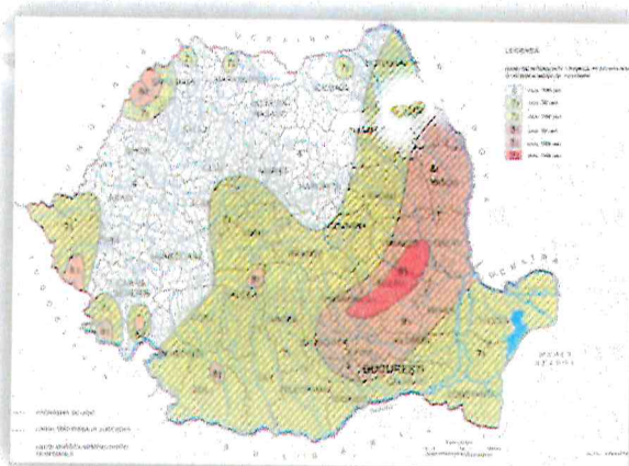
Zonarea seismică a teritoriului Romaniei.
