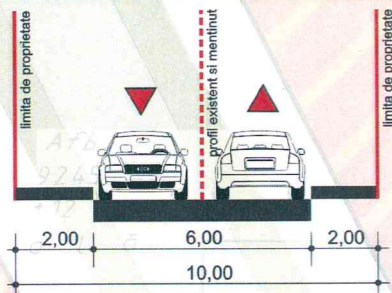
1-1. Strada Ion Cornea - Profil existent - scara 1:200
