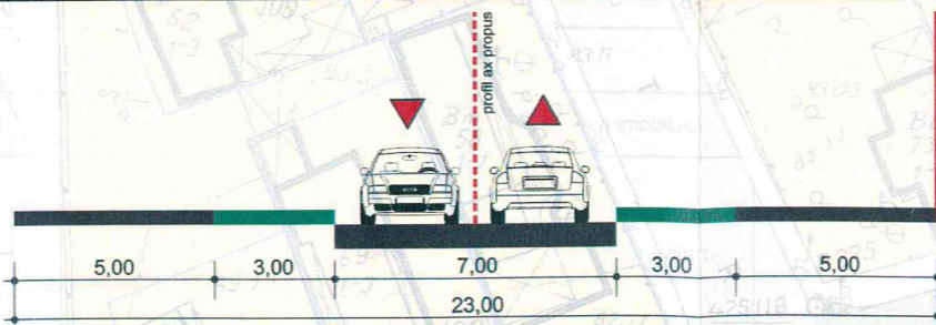
3-3. Strada propusa conform PUZ Sect. 5 - scara 1:200
